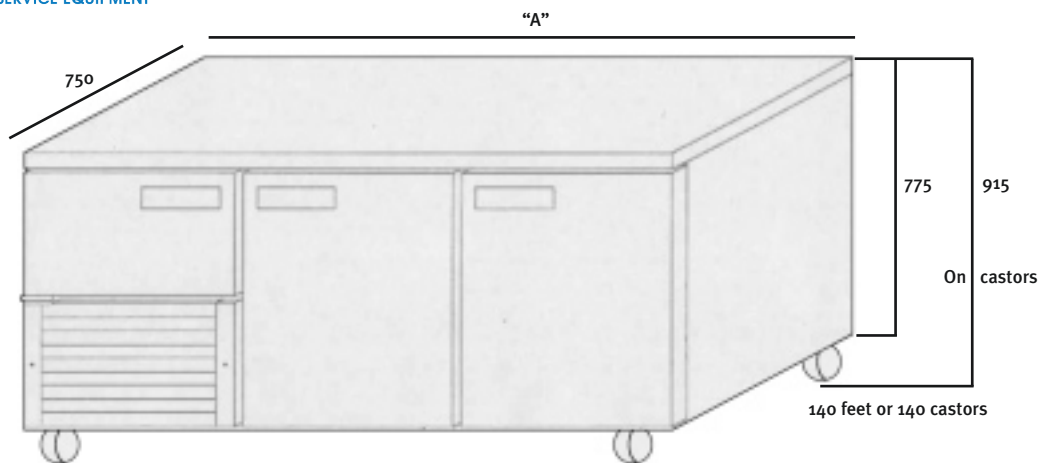
DIMENSIONS "A" - 2 1/2 DOOR - 1780mm - 3 1/2 DOOR - 2380mm
